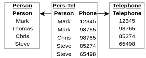
(b) Реляційна модель
